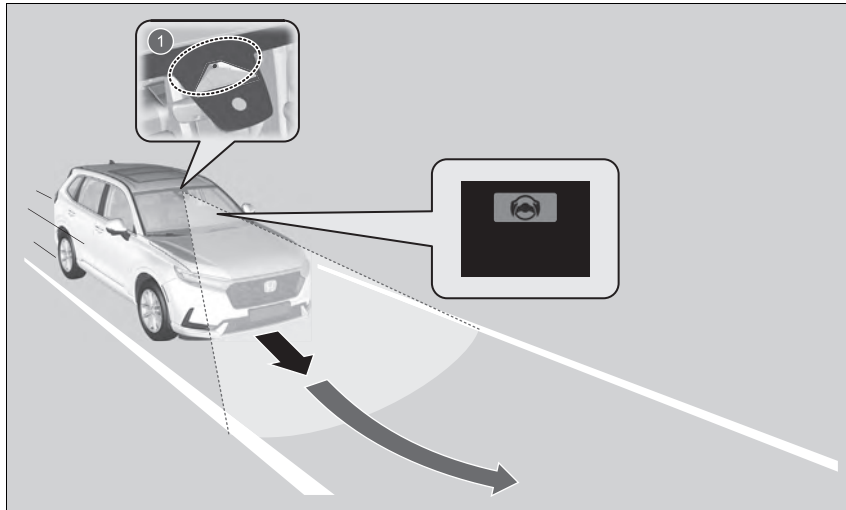
1 Caméra à capteur avant : surveille les lignes de délimitation des voies
